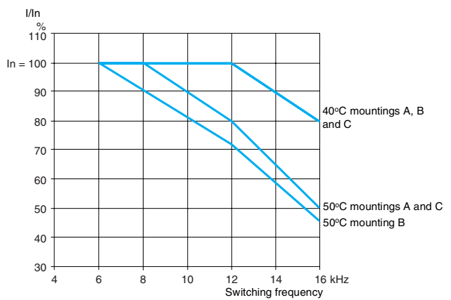
ATV 21HD37N4
