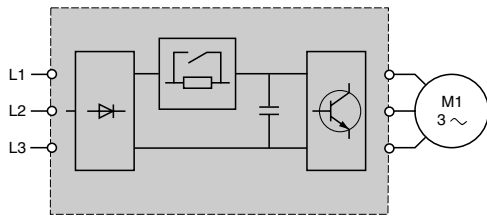
Altivar 21
