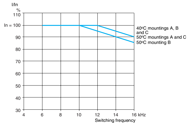
ATV 21HD15N4
