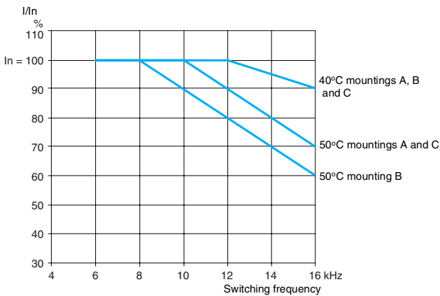
ATV 21HU55N4
