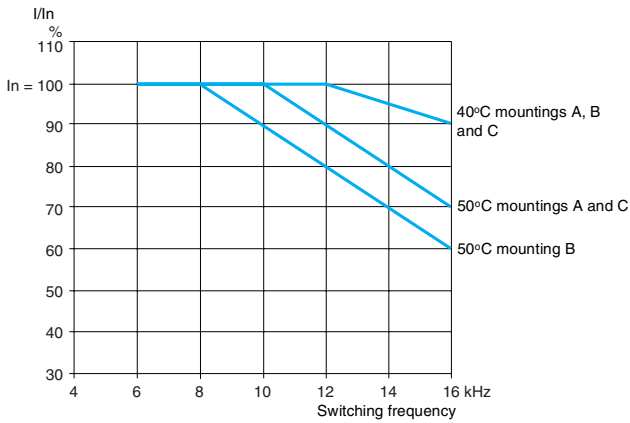
ATV 21HD18N4
