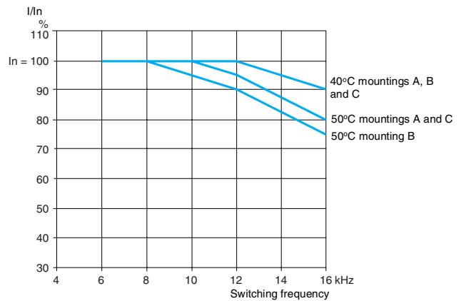
ATV 21HU40M3X
